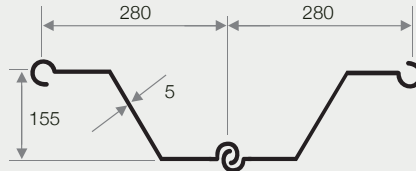
MS 280 + PILE
